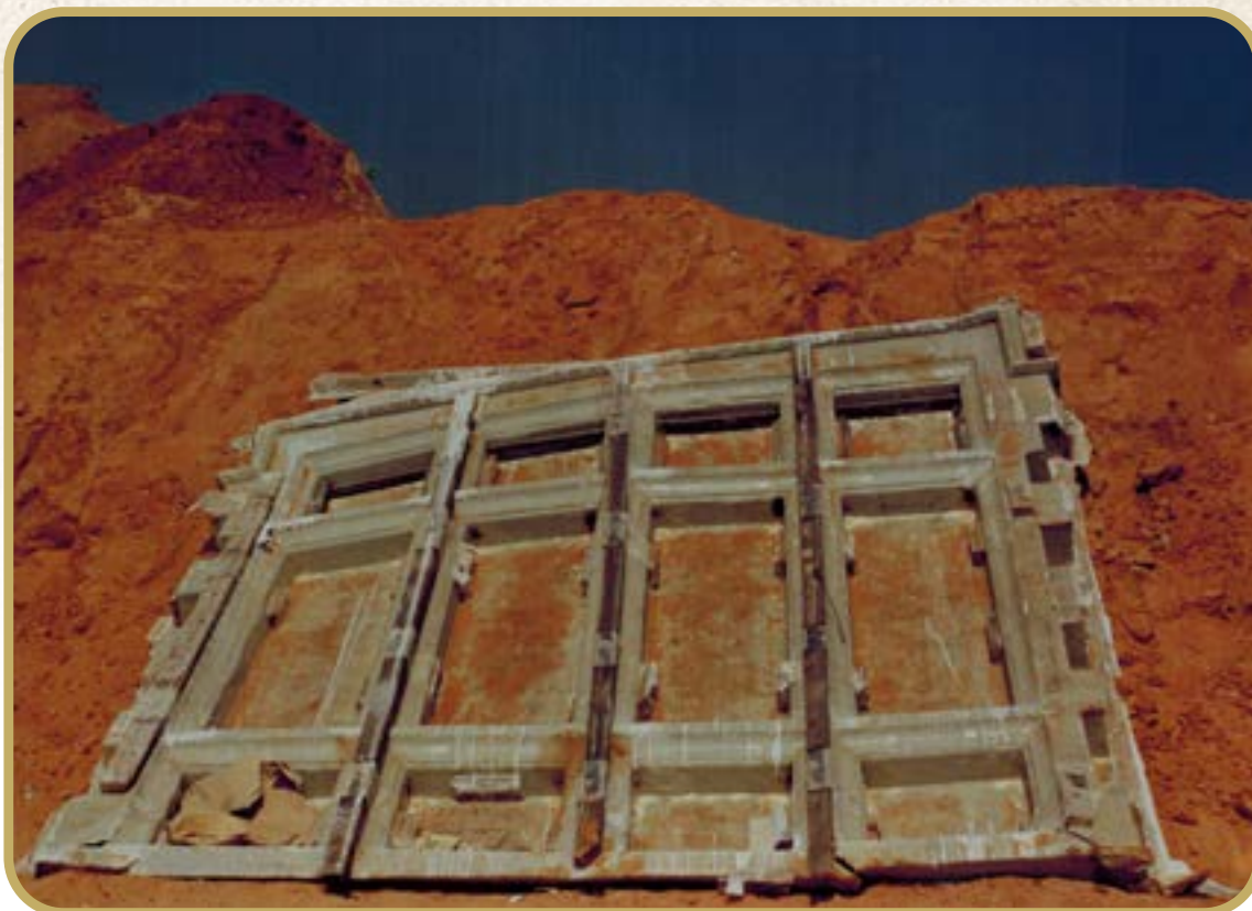
תבנית של אחד מחלונות הקומה הראשונה
